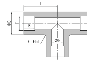
Метрическая труба
