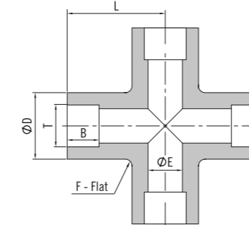
Дюймовая труба
